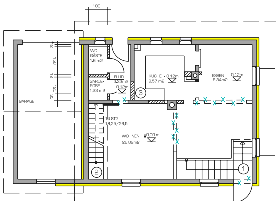
GRUNDRISS EG
