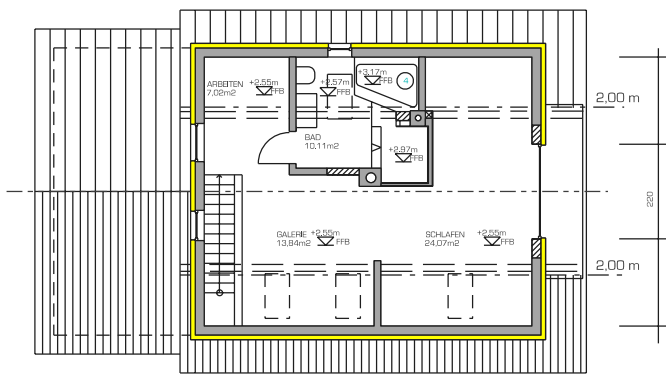
GRUNDRISS DG
