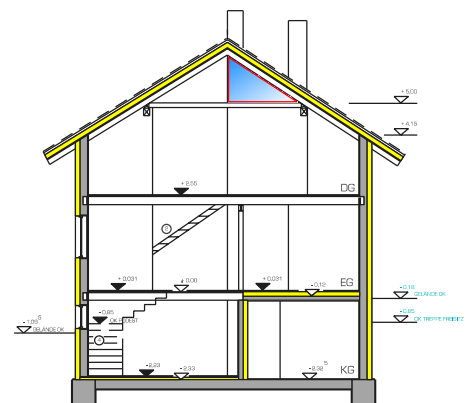
SCHNITT
